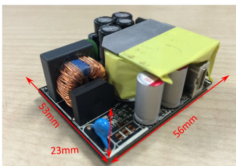
Si方案尺寸
