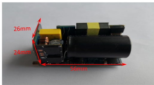
65W充電器矽與碳化鎵方案比較
